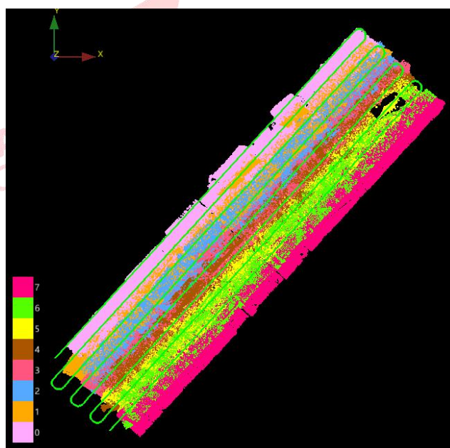
图 解算后的点云成果
