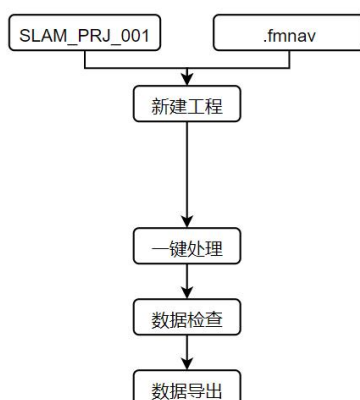
图 rtk 模式处理流程
