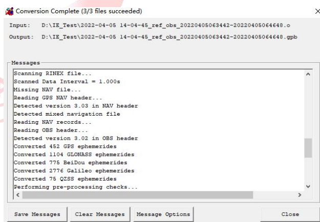
图 GPB 转换
