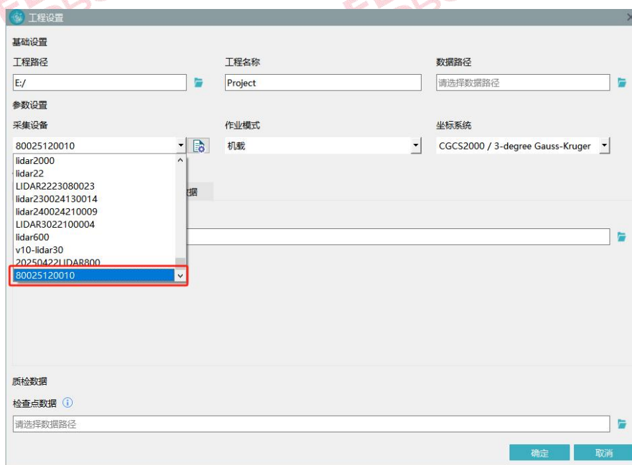
图 选择载荷
