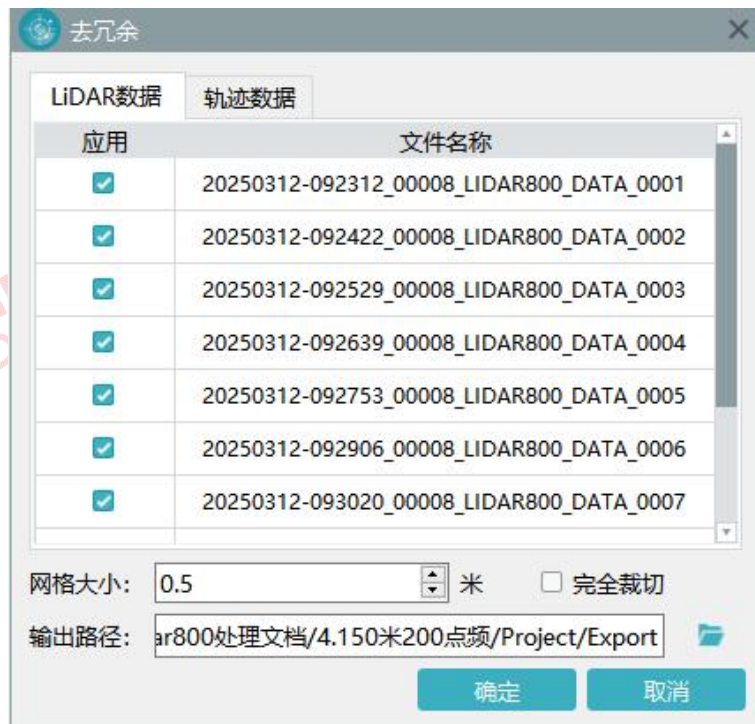
图 去冗余
