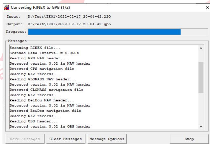
图 格式转换
