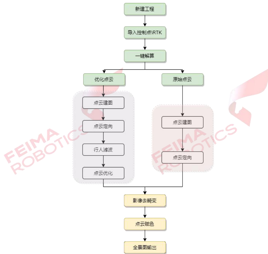
图 一键处理流程图
