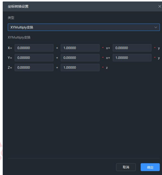
图 XYMultiply
