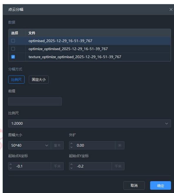
图 数据分幅
