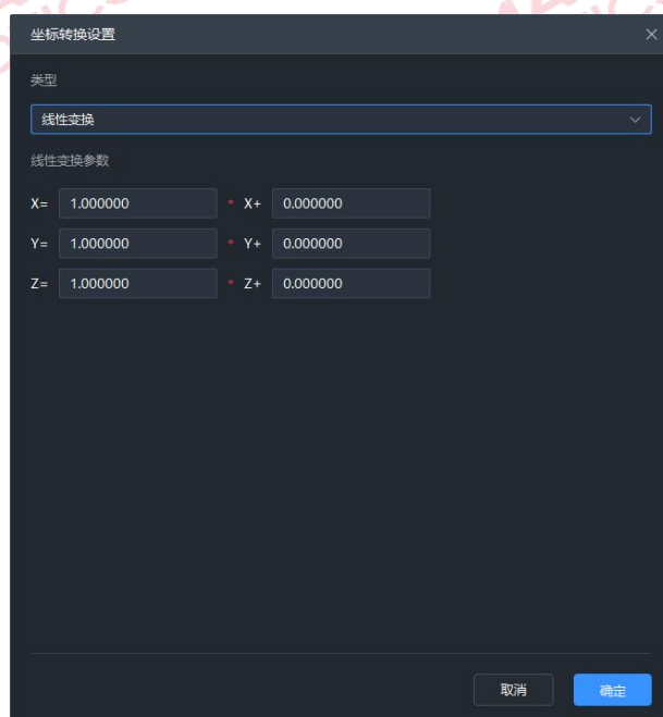
图 线性变换
