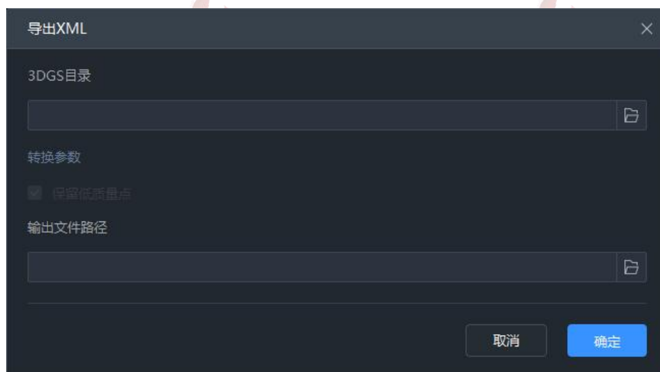
图 导出 XML
