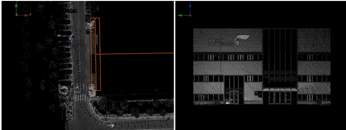
图 剖面显示
