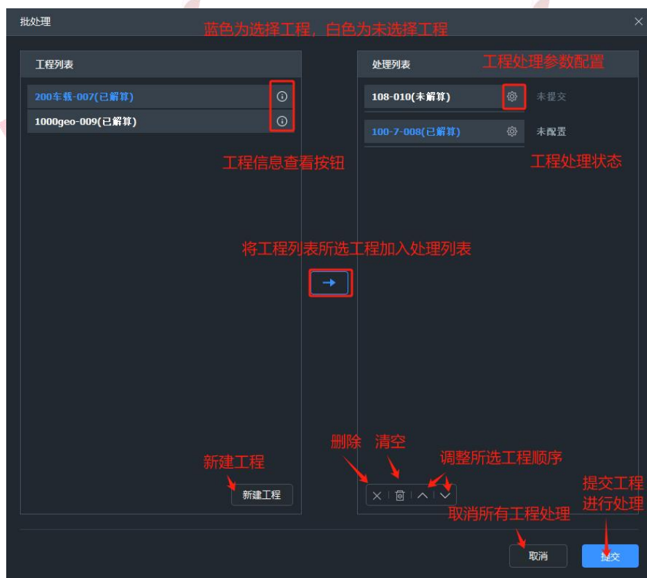
图 批处理
