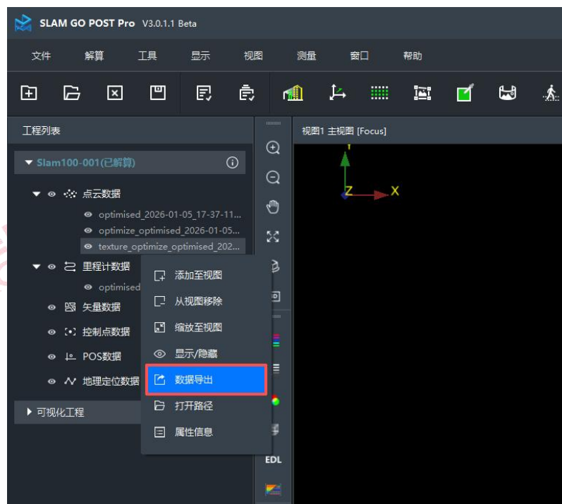
图 数据导出
