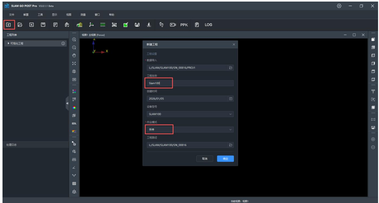
图 新建工程
