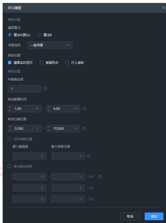
图 点云建图
