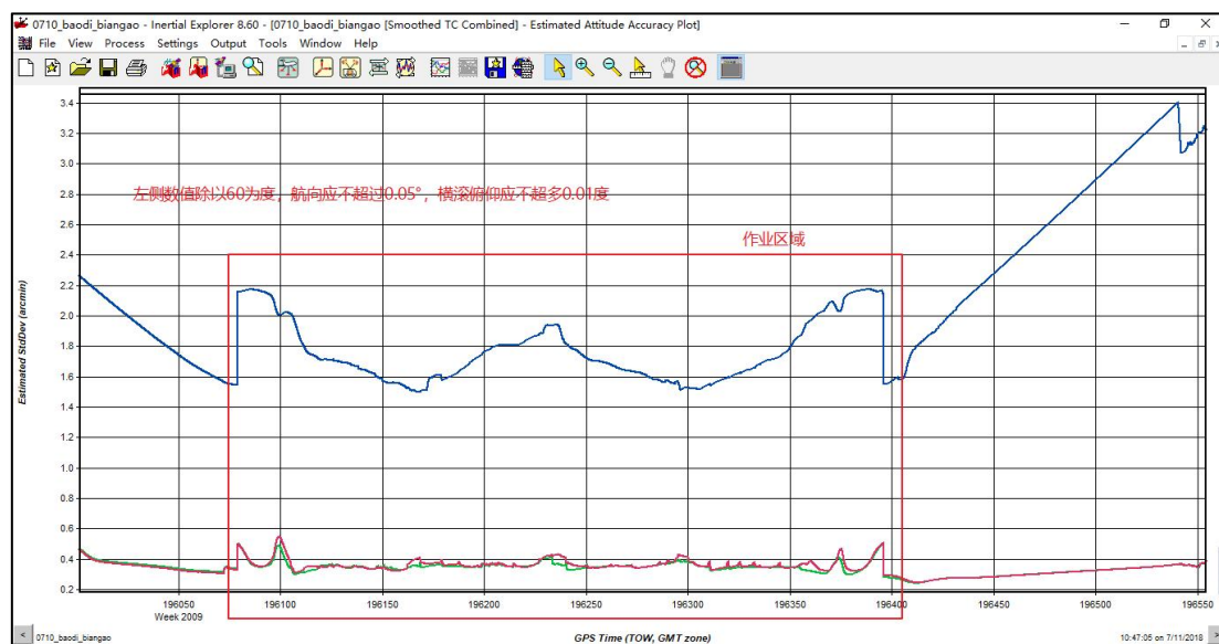
图 解算精度检查-姿态
