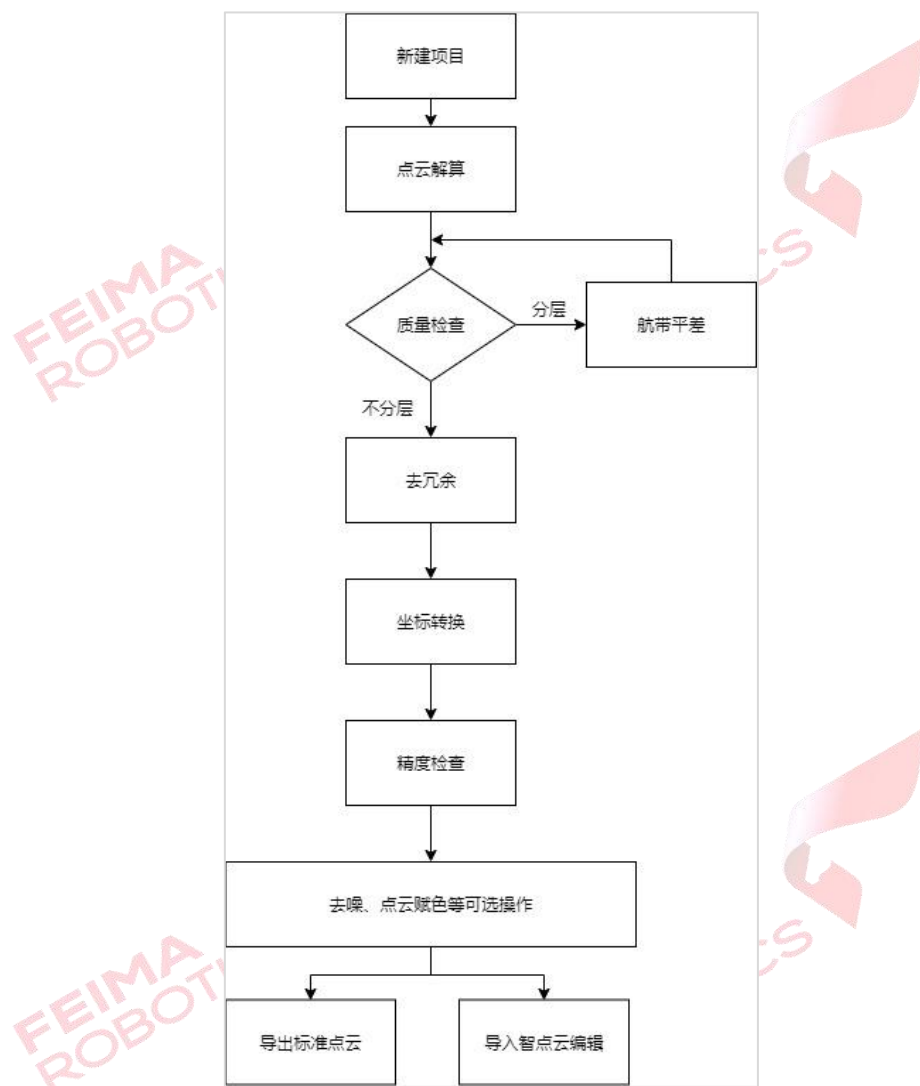
图 点云数据预处理流程图
