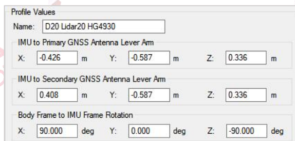
图 D-Lidar20-MEMS 版解算参数
