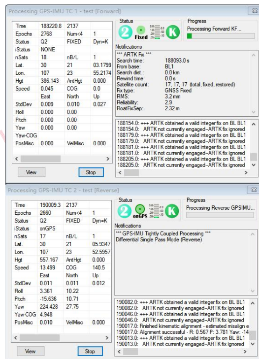
图 紧耦合解算
