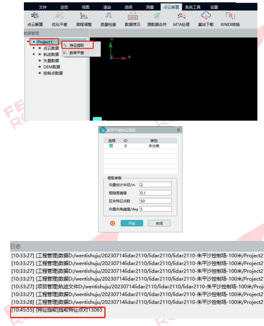
图 特征提取
