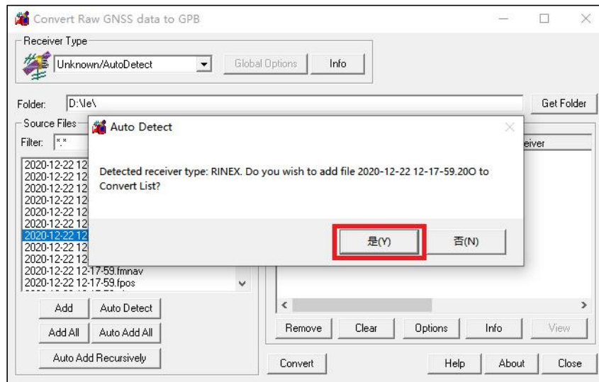
图 格式转换
