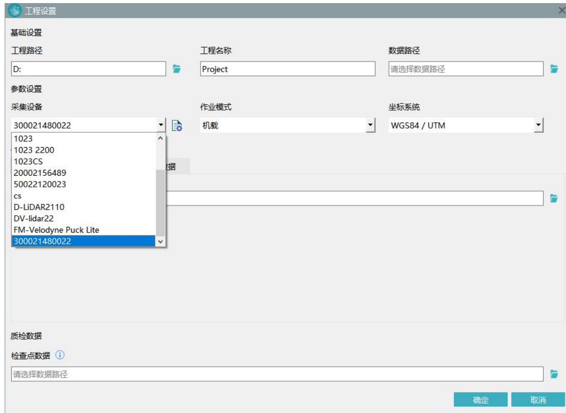
图 选择载荷
