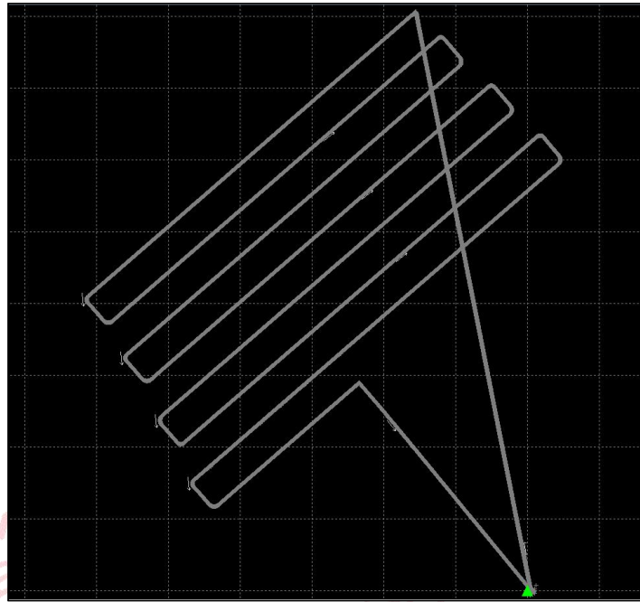
图 添加数据
