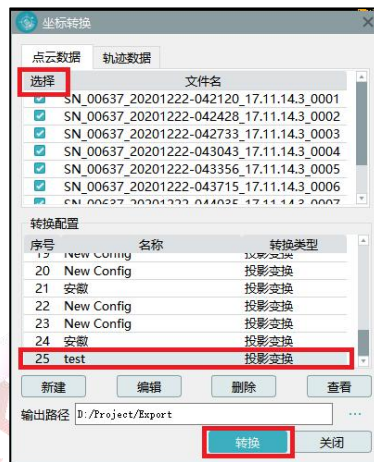
图 坐标转换
