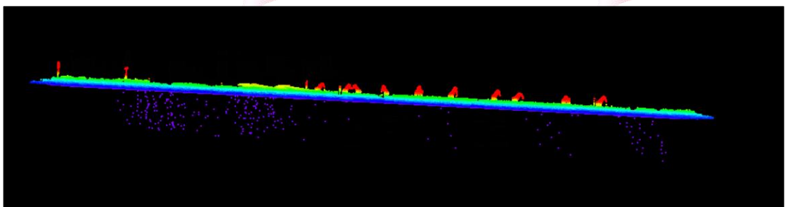
图 噪点示意
