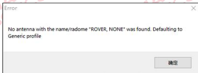
图 错误提示
