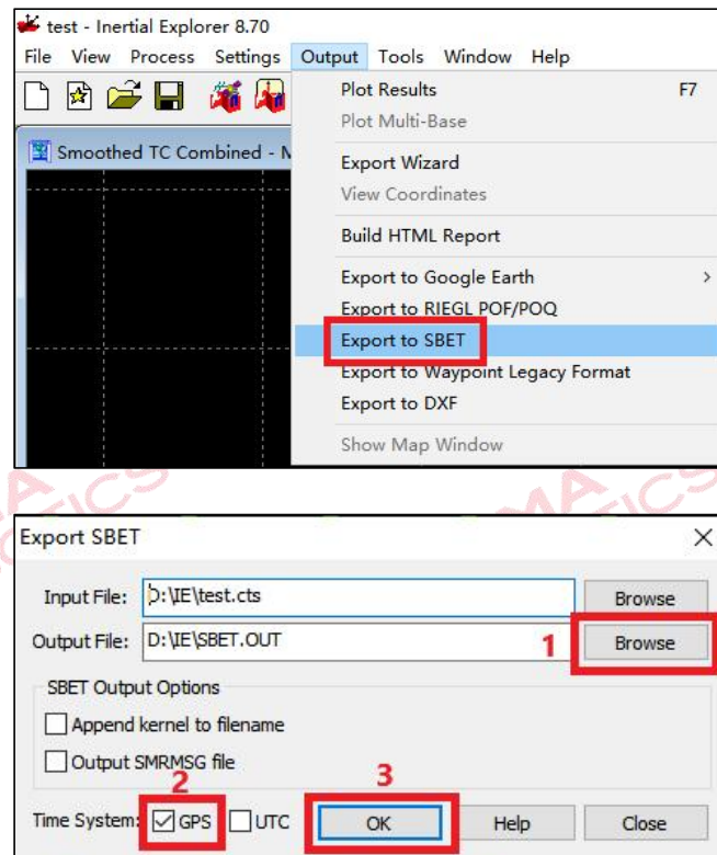
图 输出轨迹
