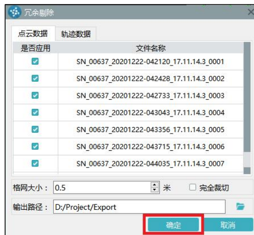
图 去冗余
