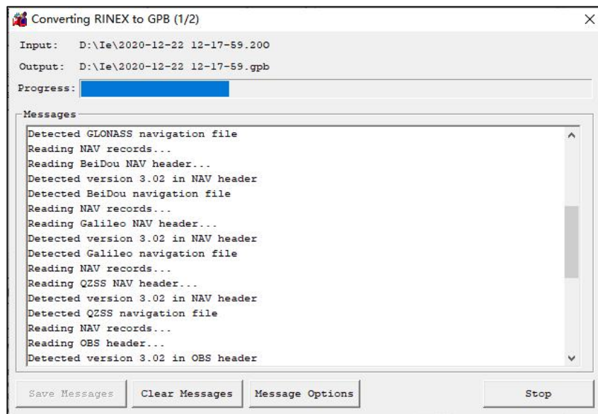
图 格式转换
