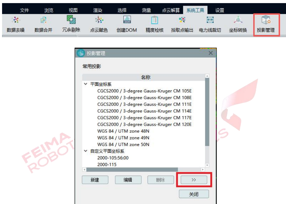
图 投影管理
