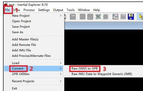
图 格式转换
