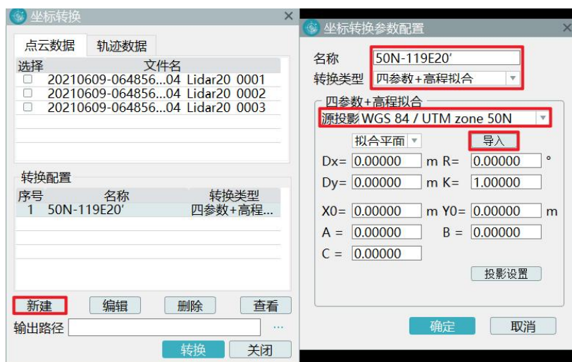
图 四参加拟合坐标转换设置
