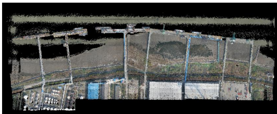
图 点云赋色
