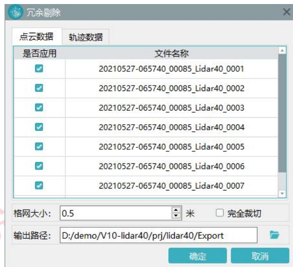
图 去冗余
