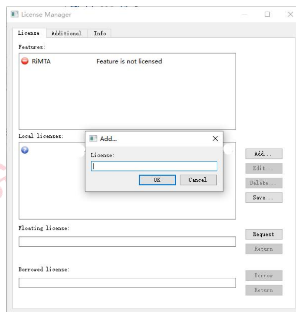
图 安装许可
