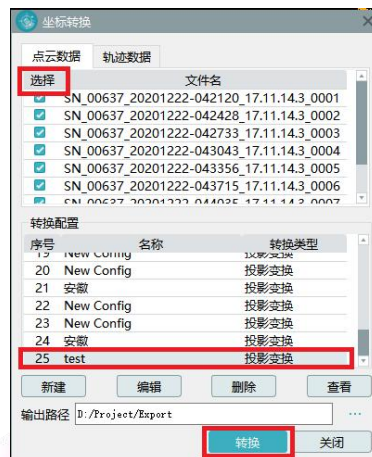
图 坐标转换
