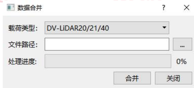
图 合并工具
