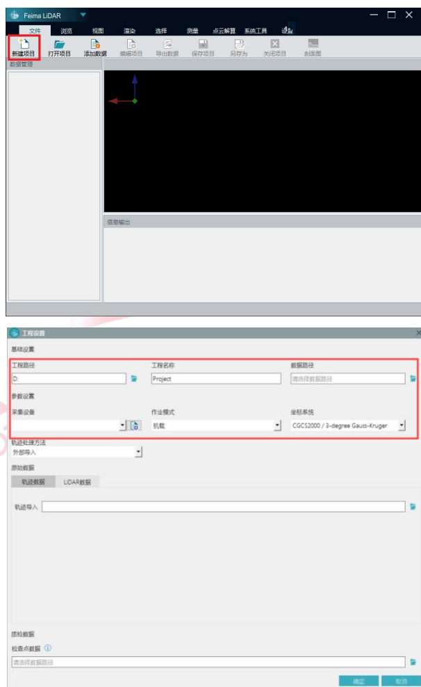
图 新建项目
