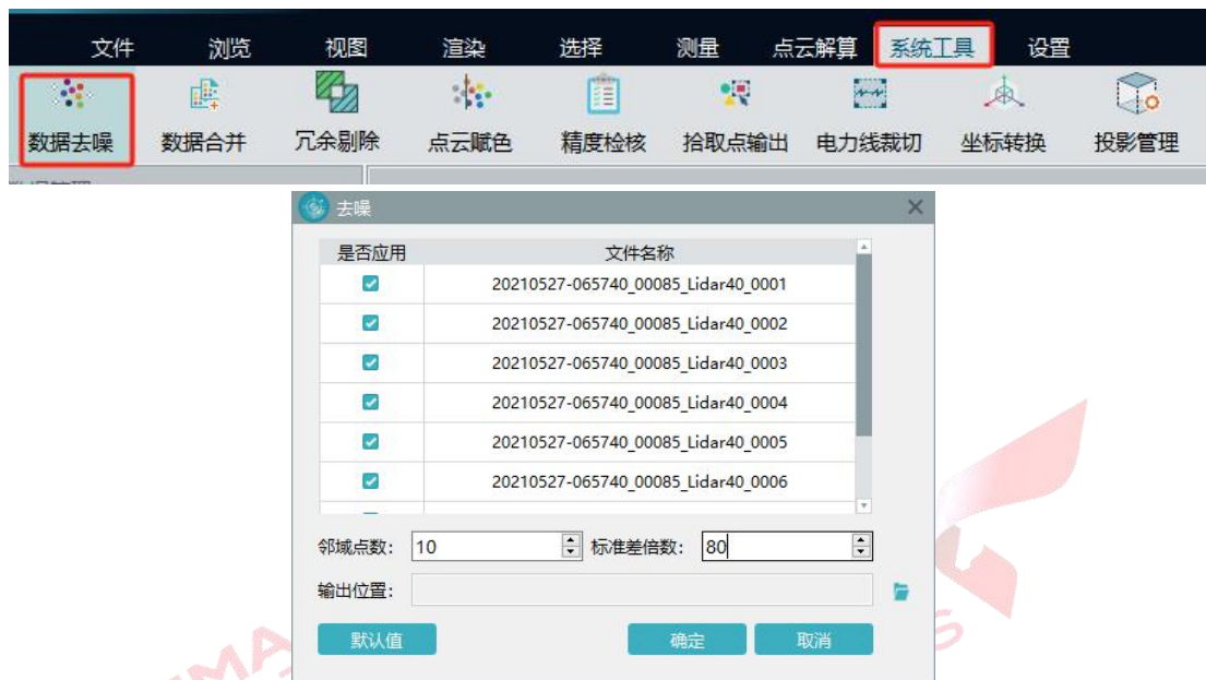
图 数据去噪
