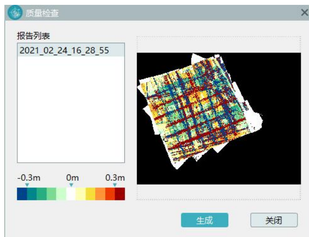
图 质量检查
