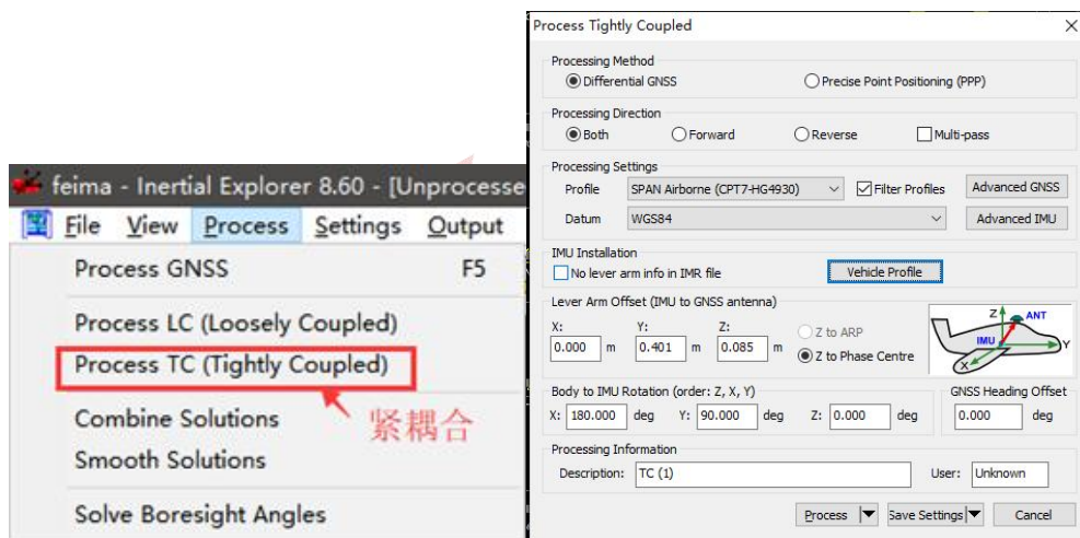
图 紧耦合解算设置
