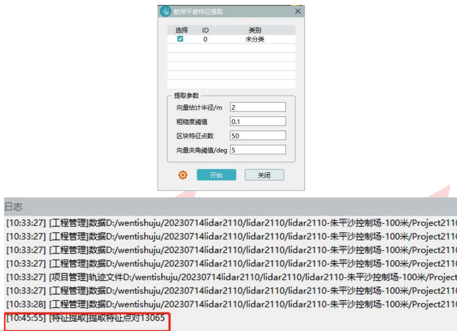
图 特征提取
