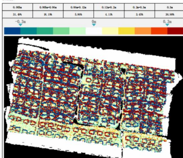
图 质量检查
