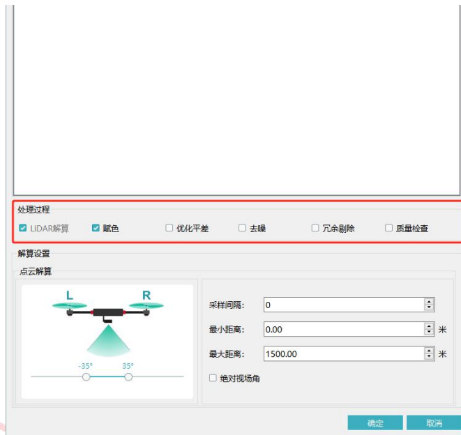
图 点云解算设置
