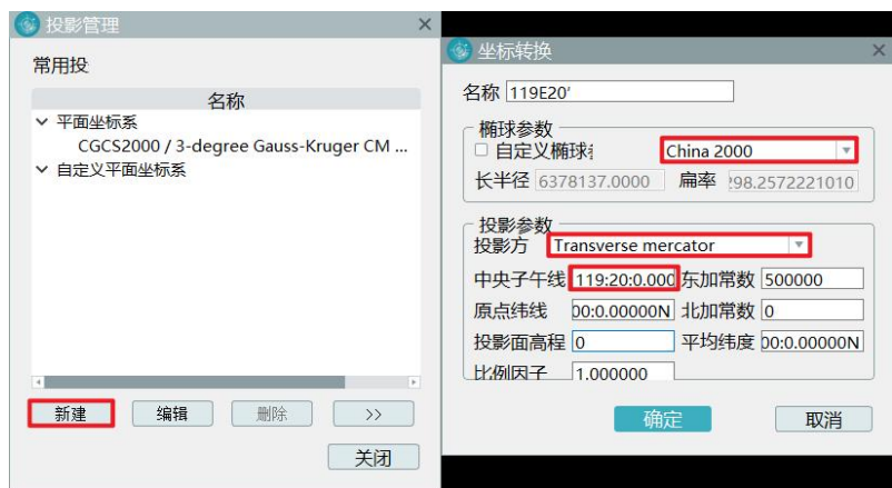
图 自定义平面坐标系统
