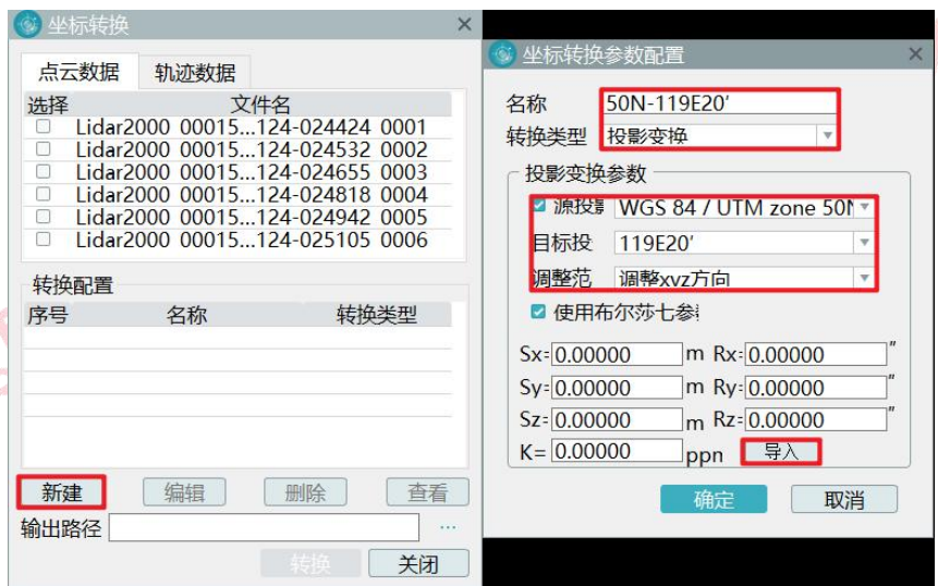
图 投影变换坐标转换设置
