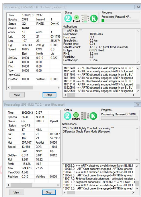
图 紧耦合解算
