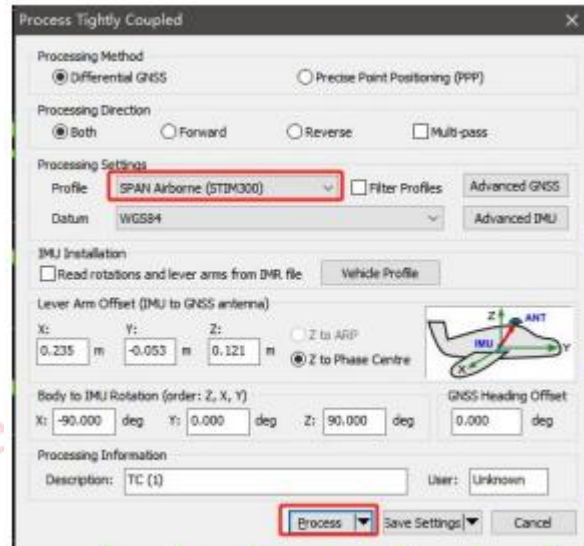
图 紧耦合解算
